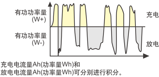
典型的重复性高速充电和放电信号
