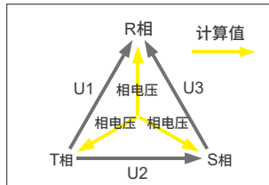
图2 三角形-星形转换
